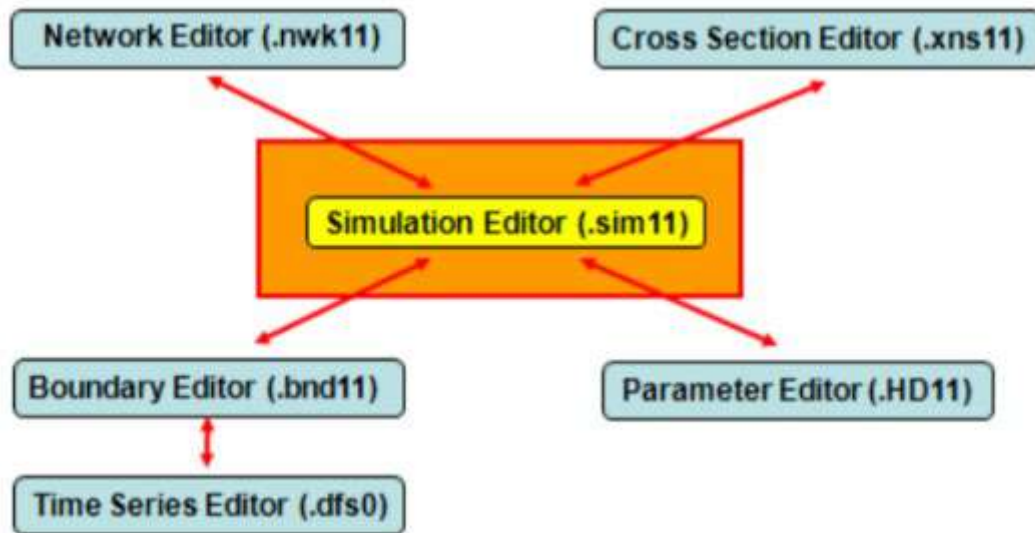
Рис. 4.11 Складові модуля конфігурації моделі MIKE11
