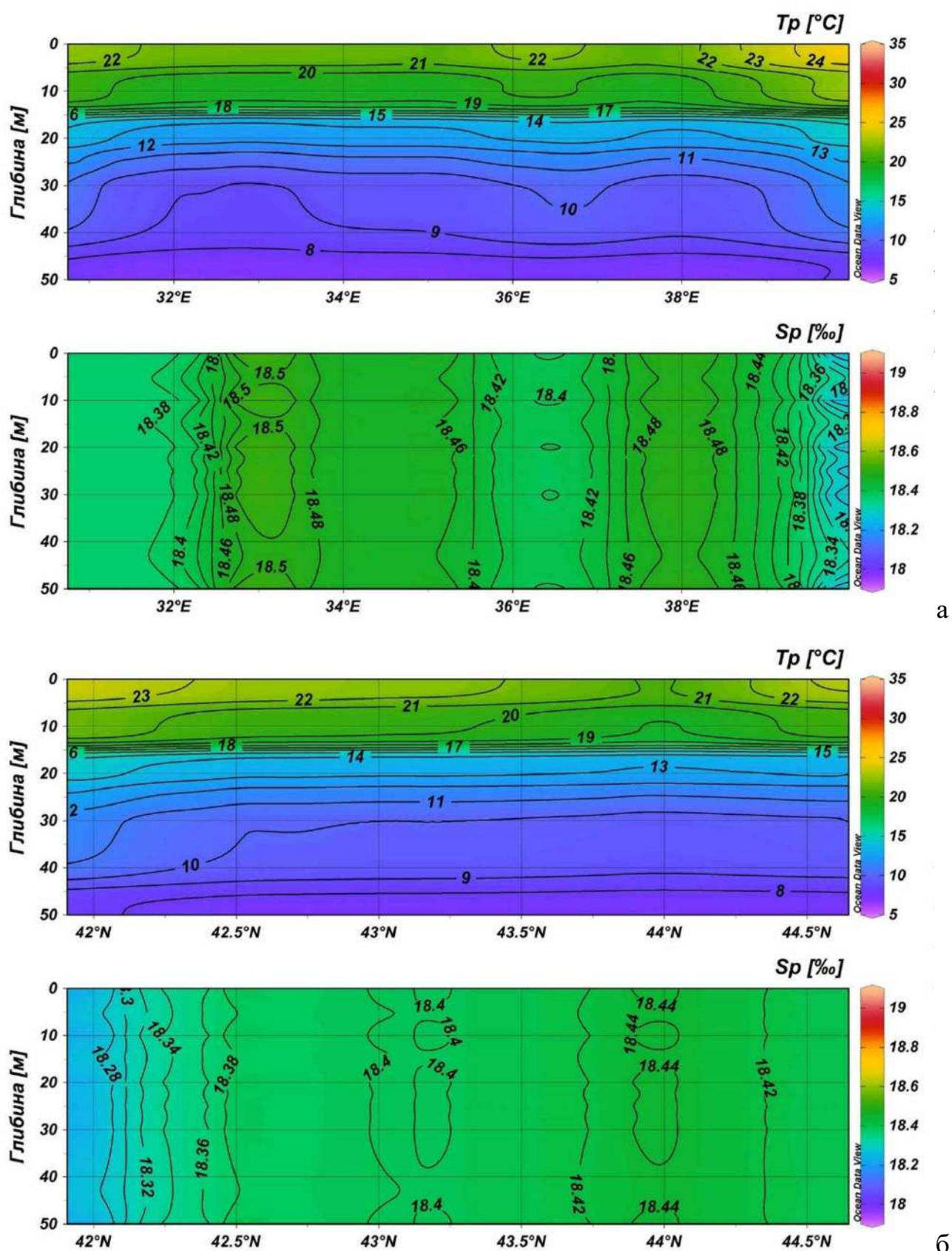
Рис. 3.12 – Розподіл розрахованої температури води ( T_p ) і солоності ( S_p ) на зональному, по широті 43,31^\circ N (а) та меридіональному, по довготі 35,77^\circ E (б) розрізах в Чорному морі для 21.09.2018р.
