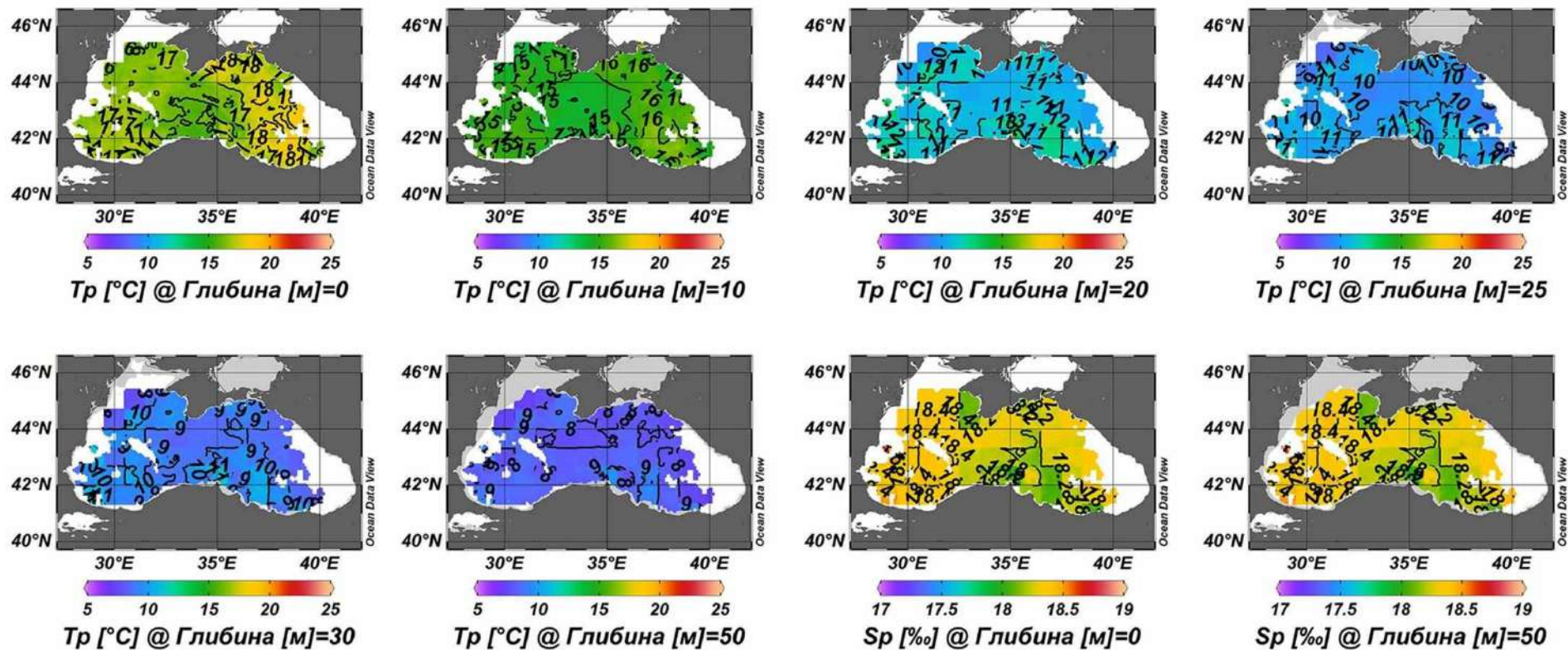
Рис. 3.3 – Карти просторового розподілу розрахованої температури води ( T_p ) на стандартних горизонтах і солоності ( S_p ) на глибині 0, 50 м в Чорному морі 15.05.2018р.
