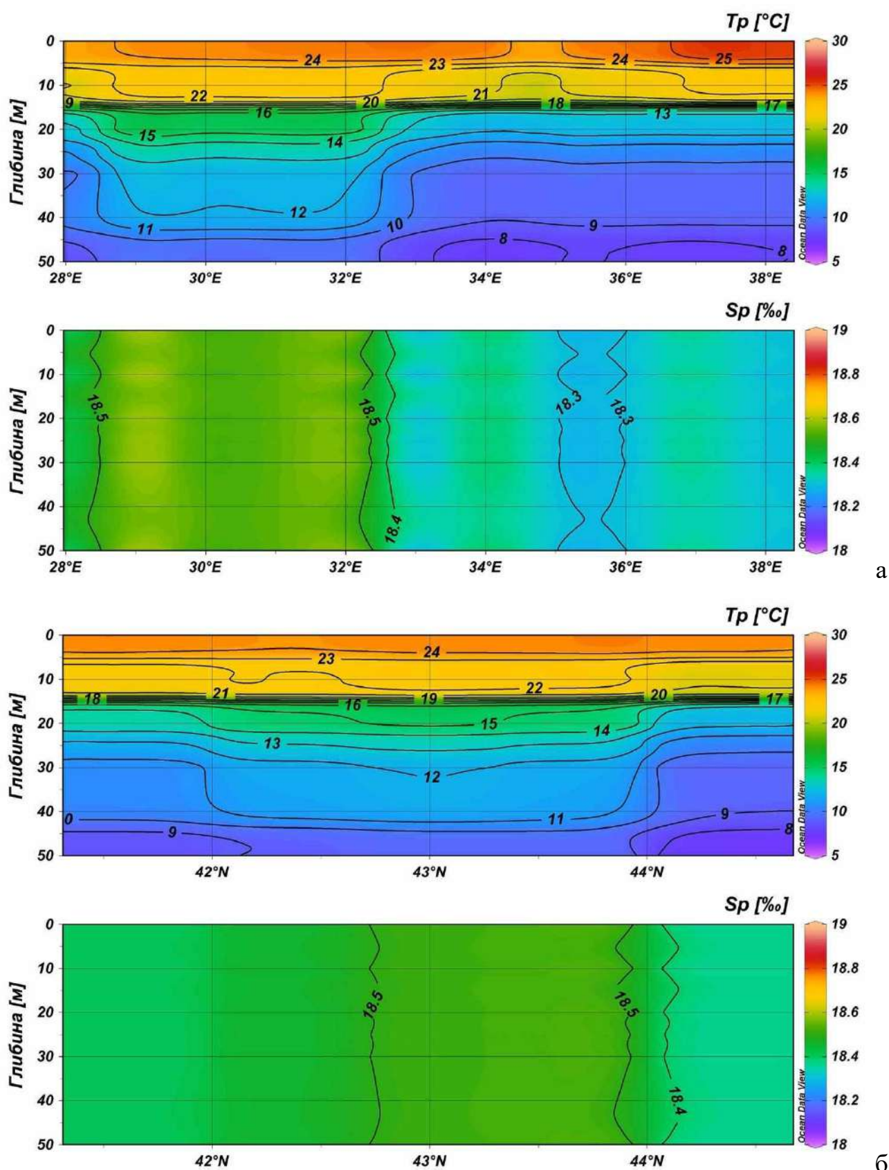
Рис. 3.6 – Розподіл розрахованої температури води ( T_p ) і солоності ( S_p ) на зональному, по широті 43,00^\circ \text{N} (а) та меридіональному, по довготі 30,40^\circ \text{E} (б) розрізах в Чорному морі для 21.06.2018р.
