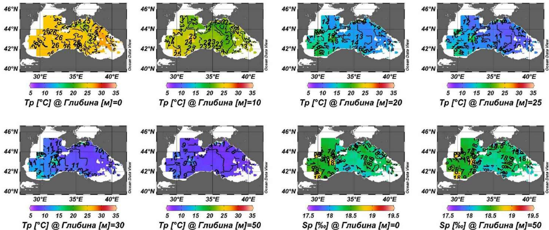
Рис. 3.9 – Карти просторового розподілу розрахованої температури води ( T_p ) на стандартних горизонтах і солоності ( S_p ) на глибині 0, 50 м в Чорному морі 23.08.2018р.
