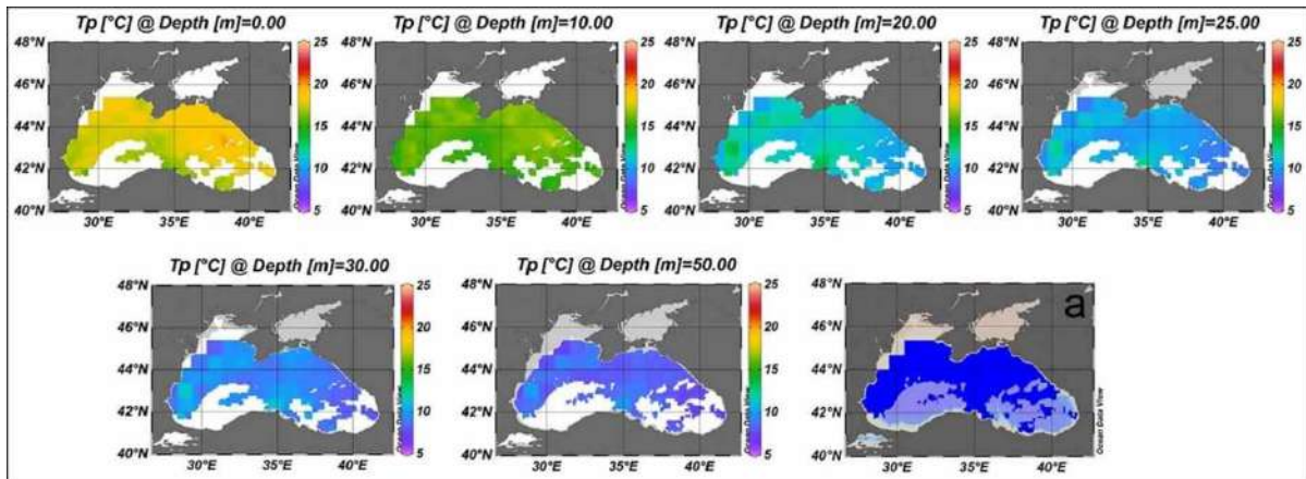
Рис. 2.19 – Карти просторового розподілу розрахованої температури води ( T_p ) на стандартних горизонтах в Чорному морі 30.05.2017г. Карта а – карта розподілу супутникових даних для розрахунків (темно-синій колір).
