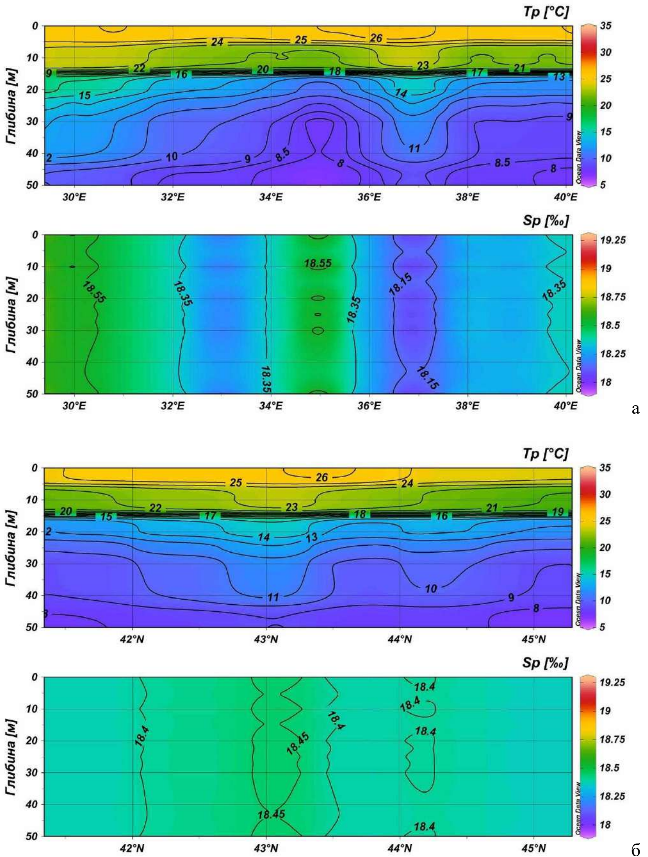
Рис. 3.8 – Розподіл розрахованої температури води ( T_p ) і солоності ( S_p ) на зональному, по широті 43,23^\circ \text{N} (а) та меридіональному, по довготі 30,85^\circ \text{E} (б) розрізах в Чорному морі для 08.07.2018р.
