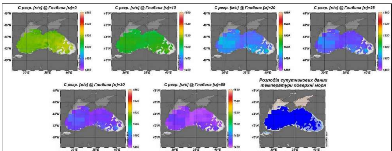
Рис. 2.31 – Карти просторового розподілу розрахованої швидкості звуку ( C_{спр.} ) на стандартних горизонтах в Чорному морі 21.06.2018р. [8]
