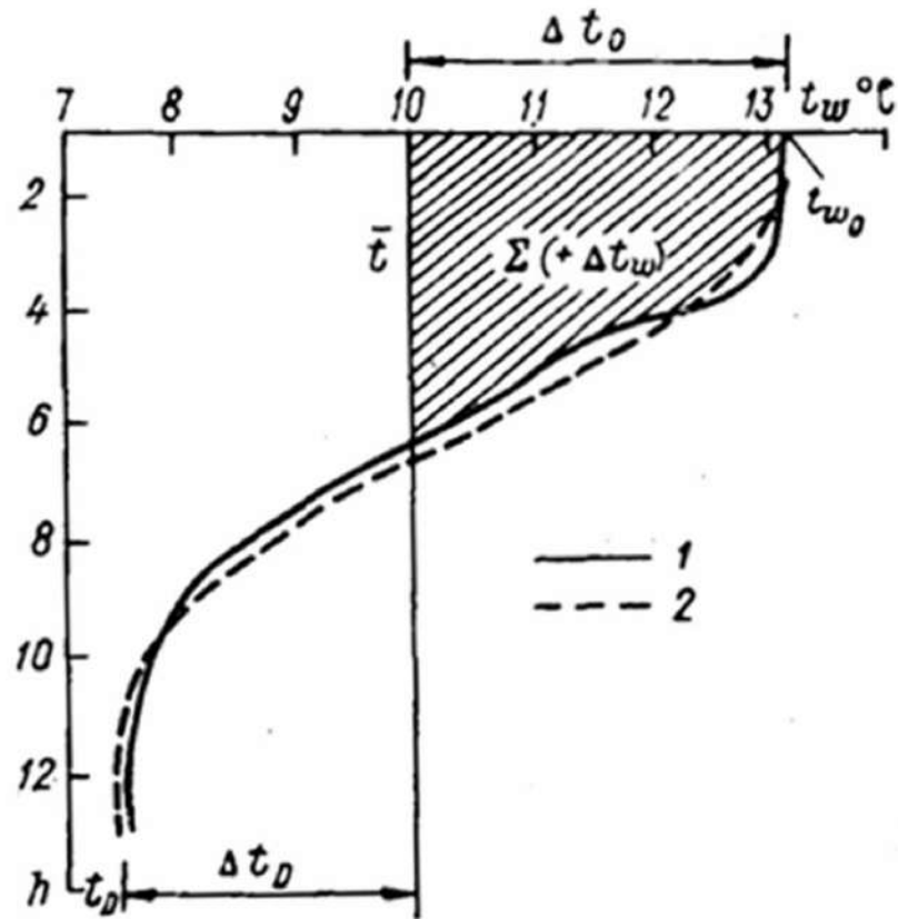
Рис. 2.4 – Параметри кривої розподілу температури води за (t_0, t_{cp}, \Sigma(+\Delta t), t_D) , згідно [53, 73, 114]
